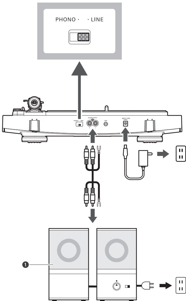
1 Aktivlautsprecher
